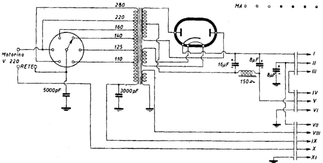
PEBA RADIO (Pertusati) - Mod. FM/106. Parte alimentatrice.
